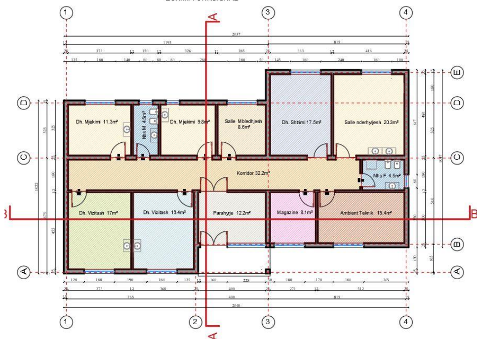
Figura 11. Planimetria e propozuar
