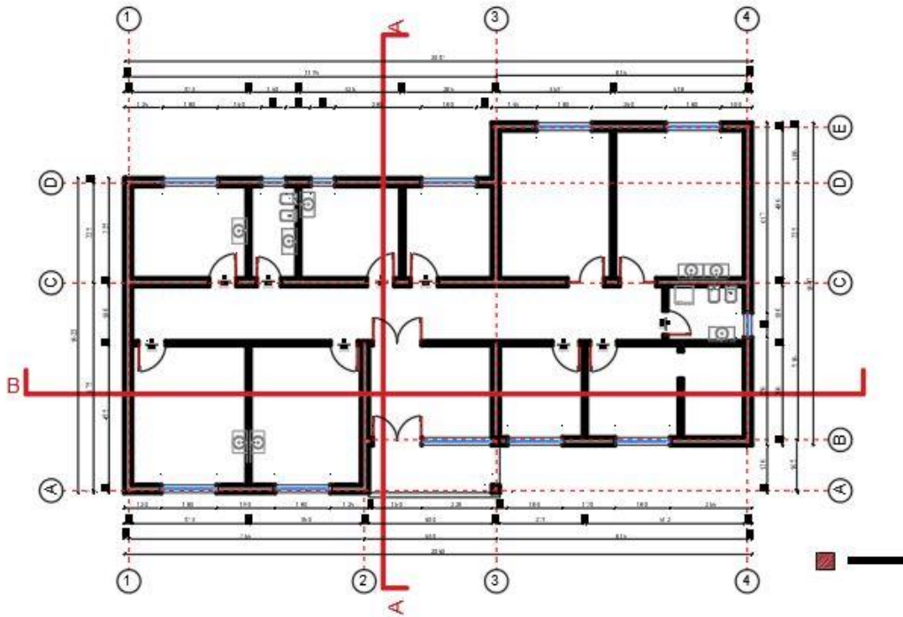
Figura 6. Planimetria e gjendjes ekzistuese
