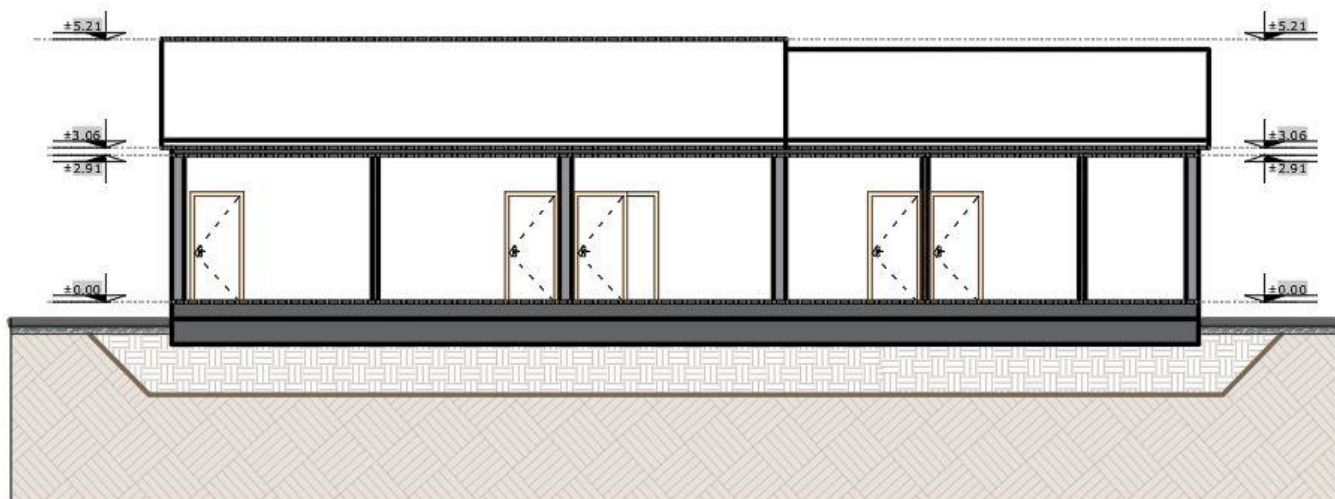
Figura 13. Prerja A-A
